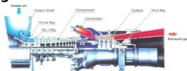
Sistema de cogeneración
